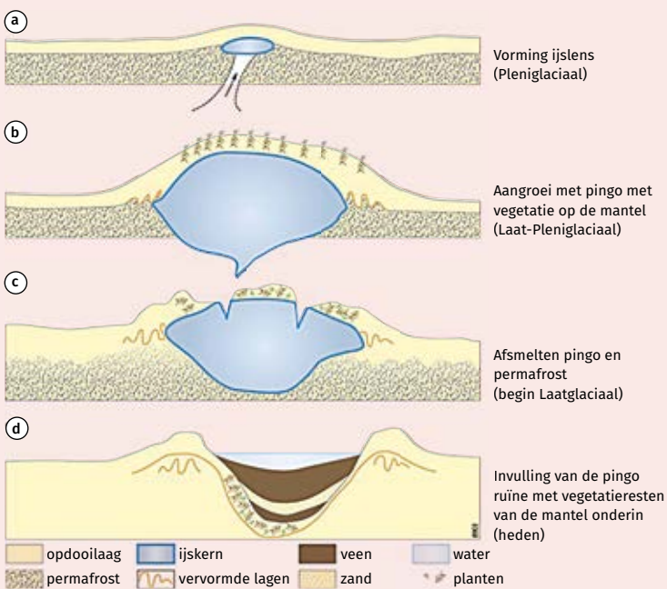
Ontstaan van een Pingo en Pingo ruïne Bron | Wim Hoek, Landschapsbeheer Drenthe
