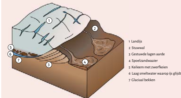
Vorming van een stuwwal en glaciaal bekken door landijs Bron | Naturalis
